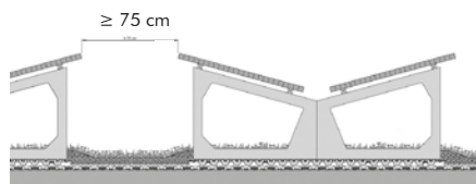
Tipo de subestructura "a dos aguas"
