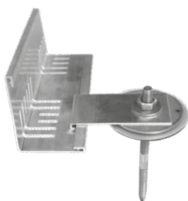
Pieza de fijación para perfil de separación KL combinada con LF 150
