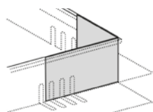
Formación de esquina interior con conector angular
