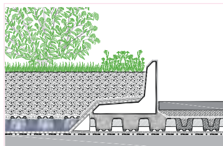
Piezas angulares de hormigón instaladas sobre fundamentos hormigonados en el elemento de drenaje Floradrain® FD 60 neo. Separan las zonas vegetadas de las zonas pavimentadas sin interrupciones del drenaje.
