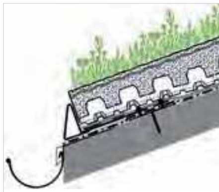
Borde perimetral con Soporte Antiempuje LF 300 en combinación con Perfil de alero TRP 140.
