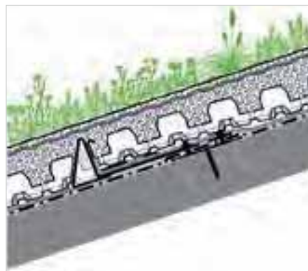
Barrera de retención, creado con el Soporte Antiempuje LF 300 y el Perfil de alero TRP 80.
