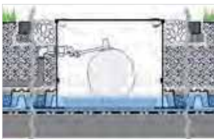
Sistema de cubierta verde intensiva con Floradrain® FD 60 neo con riego por aljibe controlado en cubiertas de 0° combinado con Autómata de riego KB 30 de ZinCo.
