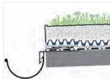
Perfil de alero DP 120
